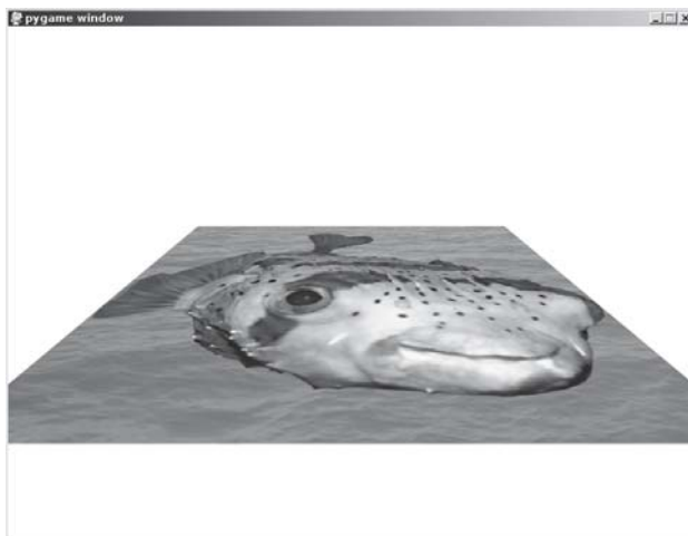
Figure 11-2. opengl.tex.py
