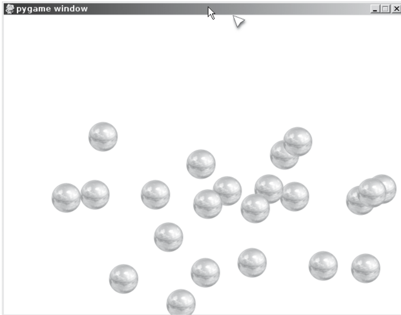
Figure 10-5. bouncesound.py
